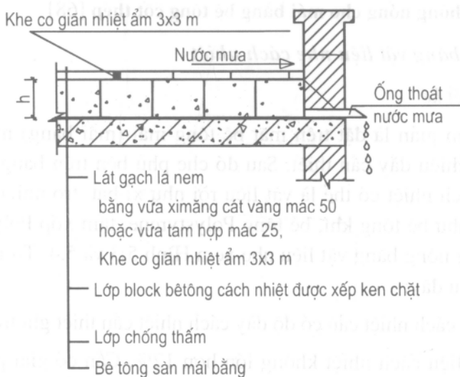
Hình 5.4. Sơ đồ chống nóng mái BTCT bằng vật liệu cách nhiệt tấm
