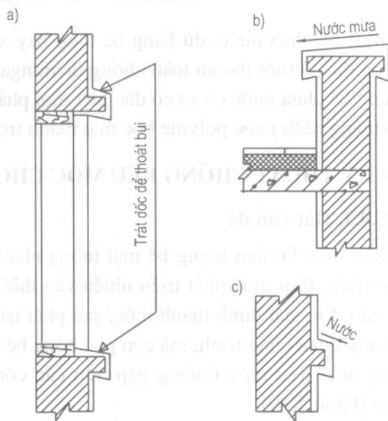
Hình 5.20. Một số chi tiết cấu tạo thoát bụi ở mặt tường ngoài công trình:
