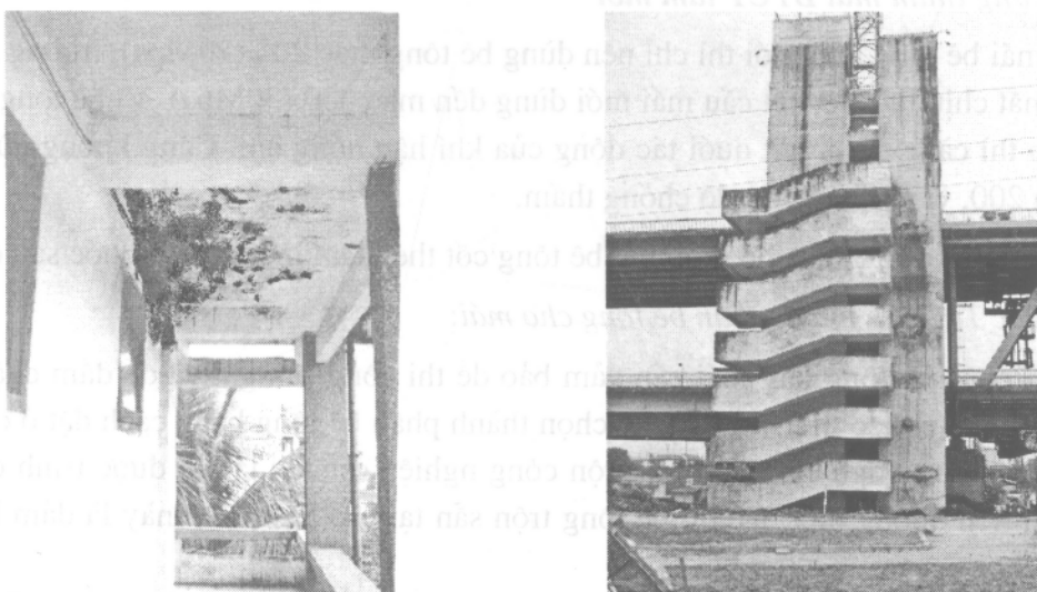
Hình 5.14. Vết thẩm sàn do bê tông không đặc chắc và vết thẩm tường do lớp xây trát trong không được chặt.
