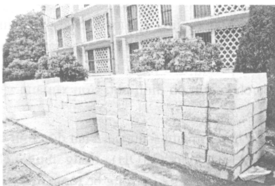
Hình 5.2. Sản phẩm Khối và tấm tường lắp nhanh từ bê tông Polystyrene [67]
