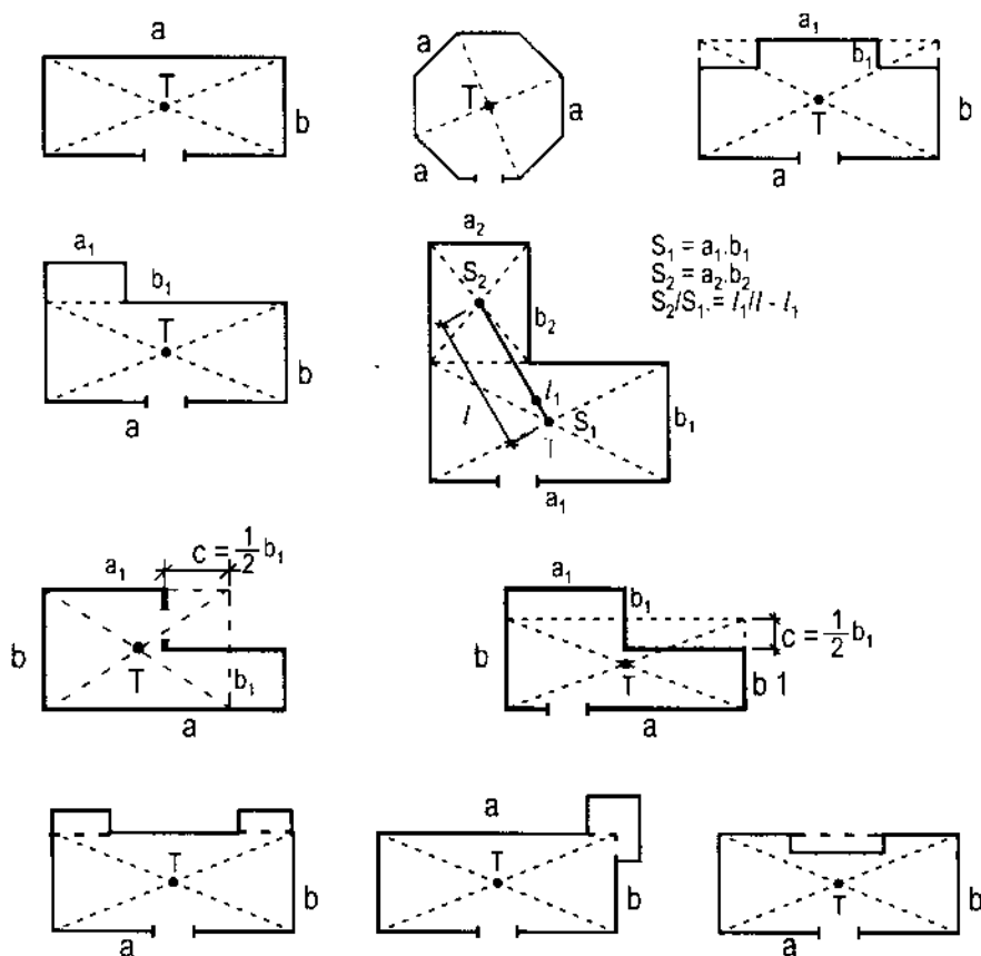
Hình 3.6. Sơ đồ nguyên tắc xác định Tâm nhà
