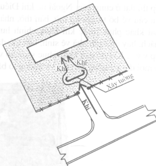
Hình 7.20. Điều chỉnh bằng tường án sơn cho nhà trực diện cuối ngõ
