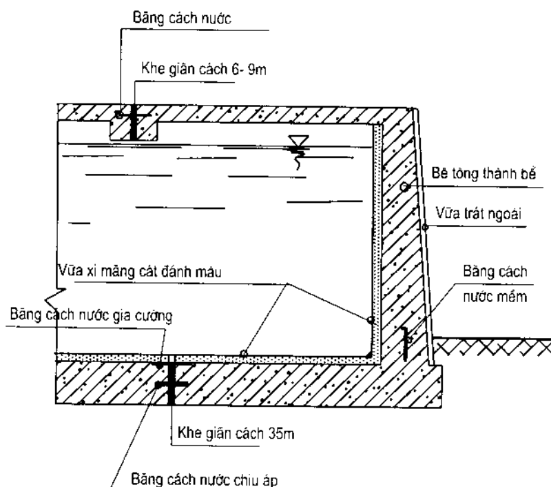
Hình 5.18. Sơ đồ cấu tạo chống thấm bể nước
