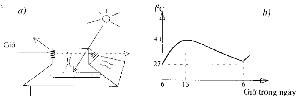
Hình 4.15. Sơ đồ hấp thụ nhiệt bức xạ mặt trời của mái BTCT dán ngói
