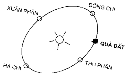
Hình 7.3. Quy đạo trái đất quay xung quanh mặt trời
